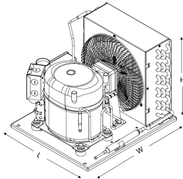
Standard FHP: TYA TYA4466YKS TYA4475YKS
